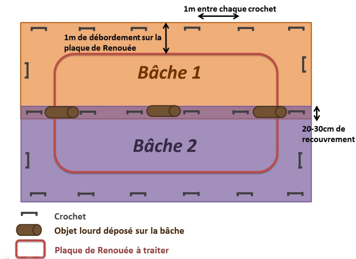
Figure 11 : Schéma de la technique du bâchage
